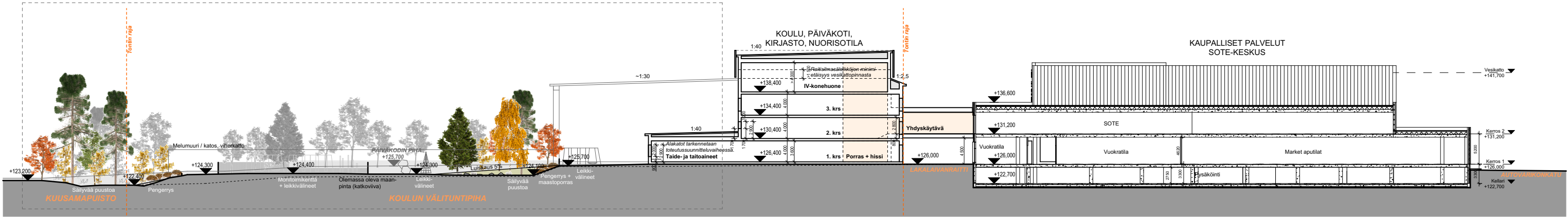
Alueleikkaus A-A
