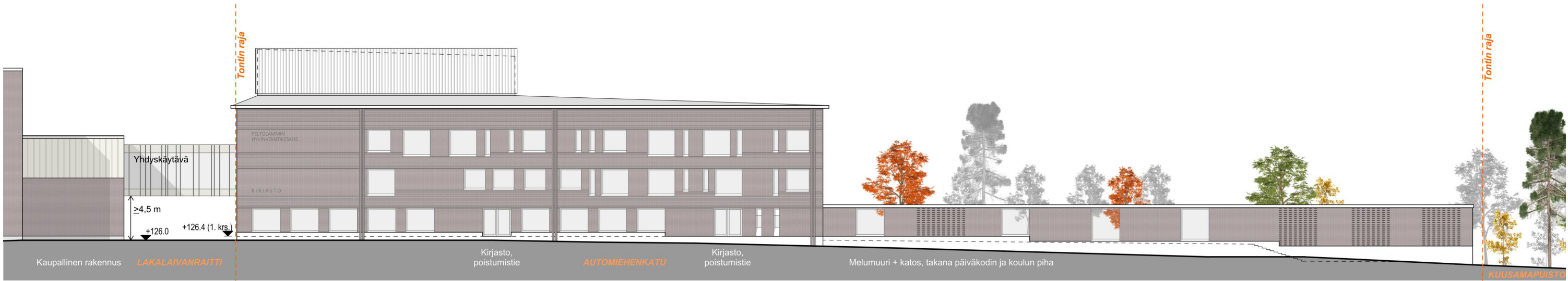
Julkisivu pohjoiseen (Automiehenkadulle)
